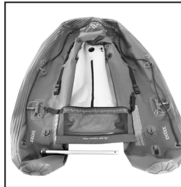
3. Desfaceți „rigla de plasă” cu marginea manșonului îndreptată spre „țeava de montare lungă din 2 piese”.
